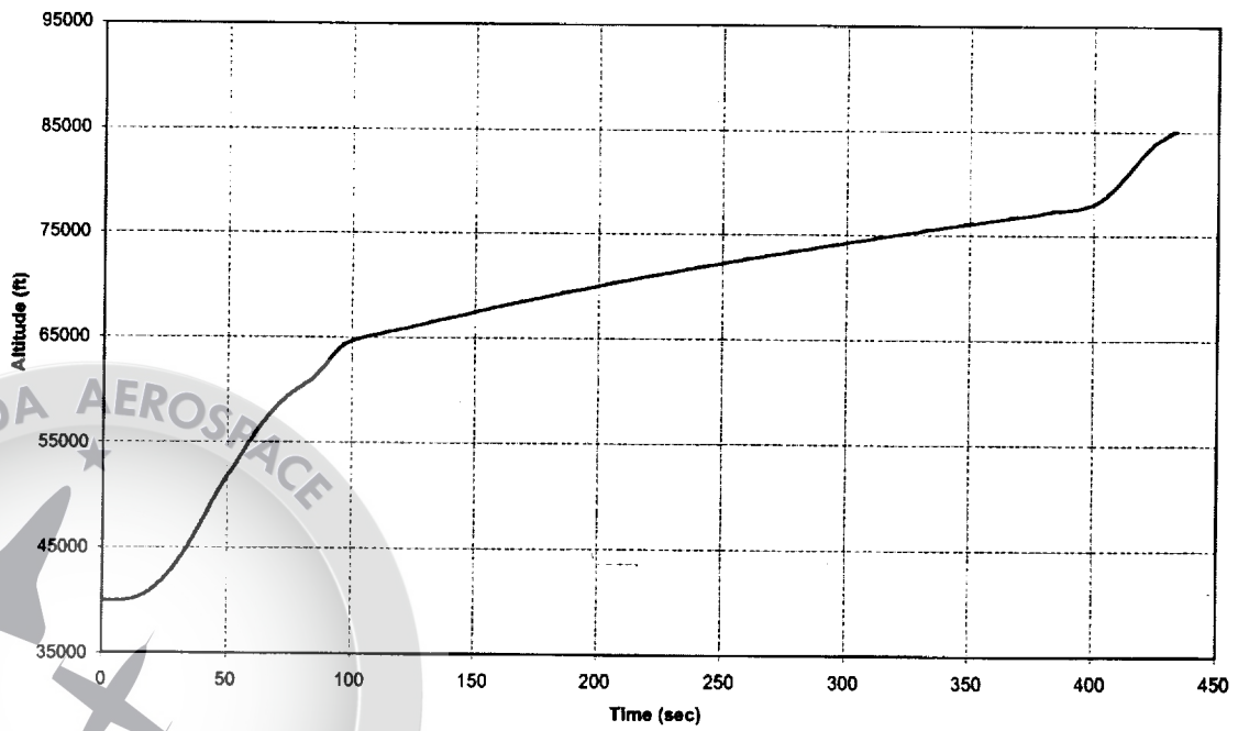
NASAE3CTLOX/ProC1 Altitude vs Time
