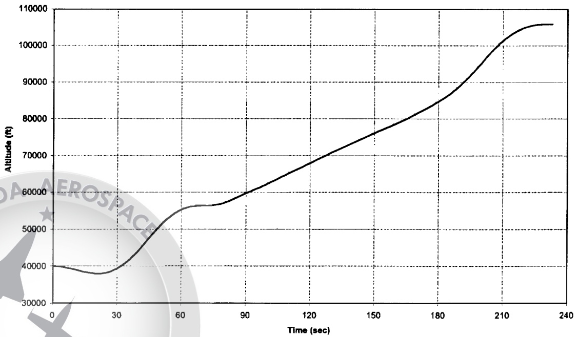
NASAE3GTLOX/JPA Altitude vs Time
