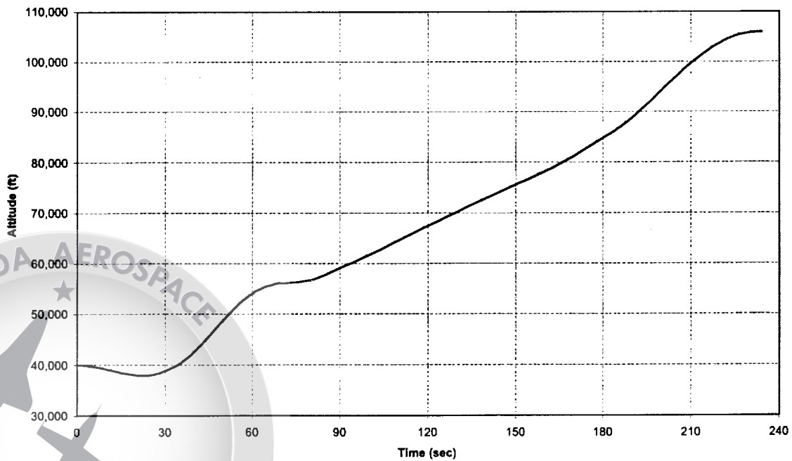
NASAE3GTLOX/PRA Altitude vs Time
